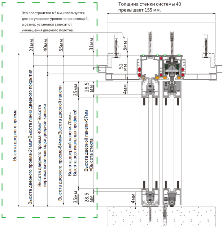
Поперечное сечение дверного проема
