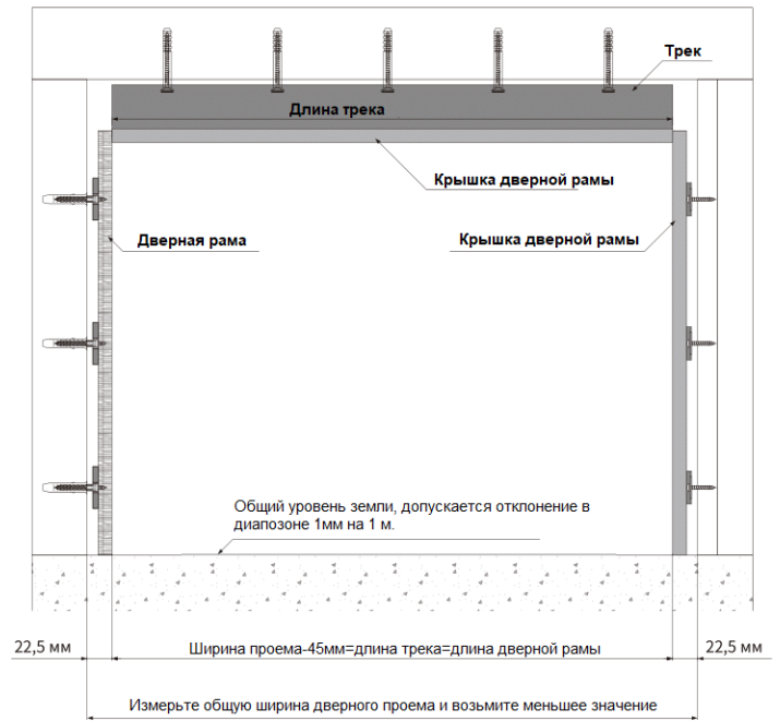
Вид дверного проема спереди
