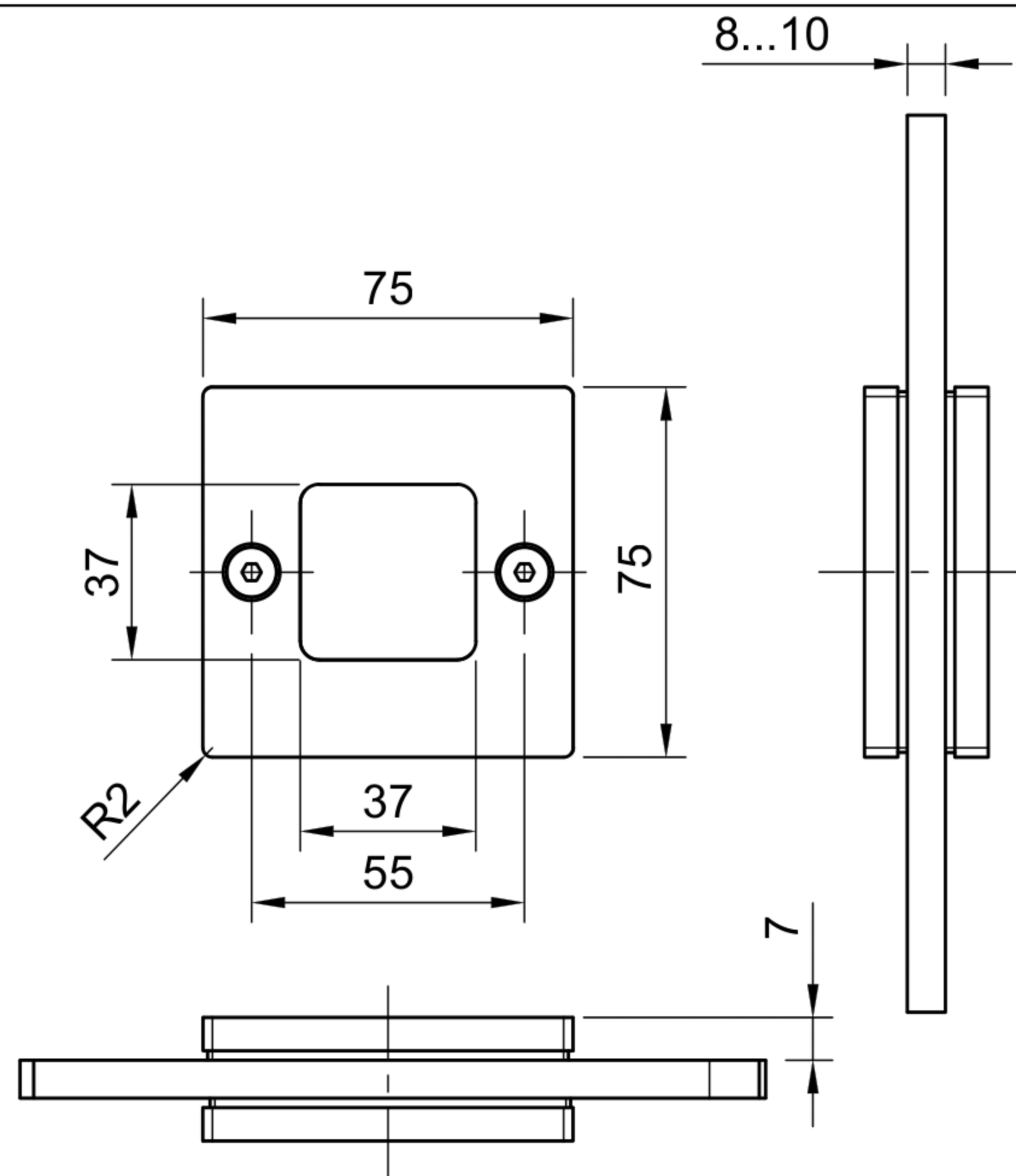
Эскиз установочных отверстий в стекле
