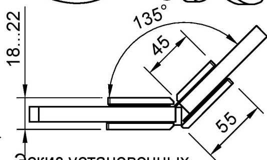
Эскиз установочных отверстий в стекле
